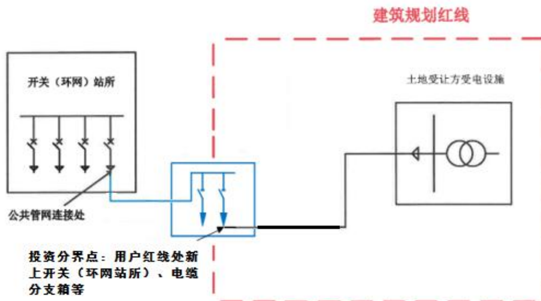
图3 从开关（环网）站所接入的高压类项目电力接入工程
